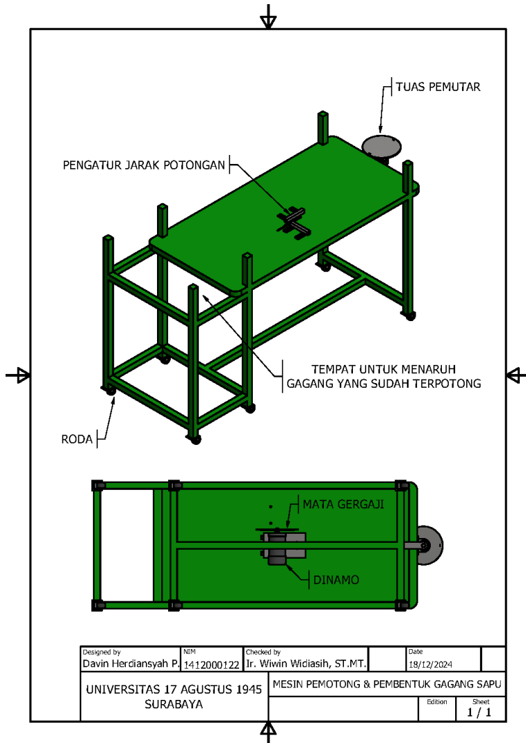
Gambar lampiran 5 Desain keseluruhan perancangan ulang alat
