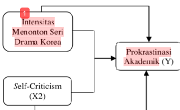
Gambar 1. Kerangka Berpikir
