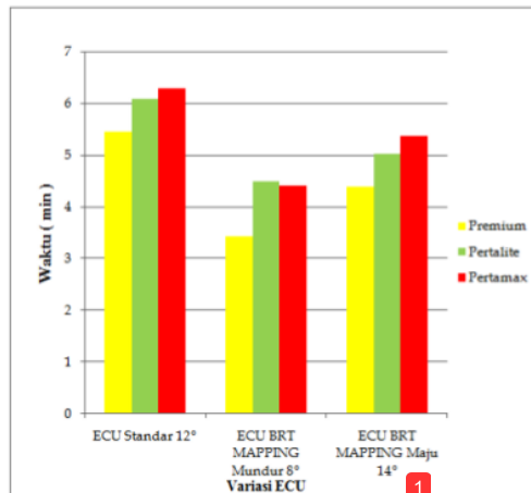
Gambar 5. Grafik Perbandingan Konsumsi Bahan Bakar
