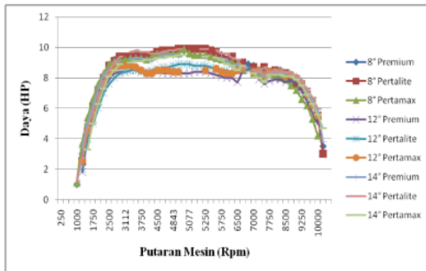
Gambar 3. Grafik daya setiap variabel terhadap Rpm
