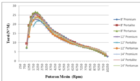
Gambar 4. Grafik torsi setiap variabel terhadap Rpm
