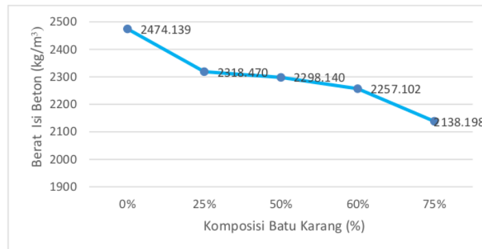
Grafik 1. Rata-Rata Berat Isi Beton Segar
