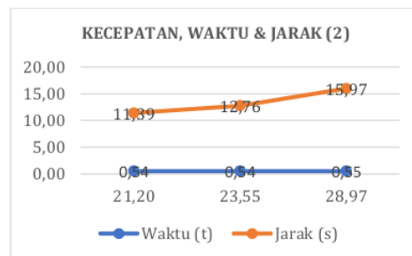
Gambar 10. Grafik Pengujian Kecepatan Konveyor 2
