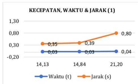
Gambar 9. Grafik Pengujian Konveyor 1
