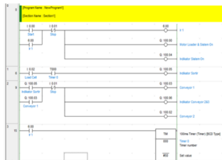
Gambar 3. Simulasi Menggunakan CX Programmer
