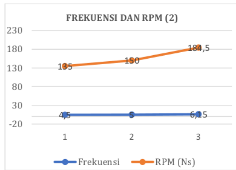
Gambar 8. Grafik Pengujian Frekuensi dan RPM Konveyor 2
