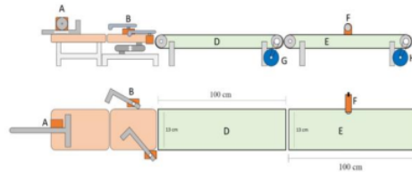
Gambar 2. Design Rancangan Konveyor
