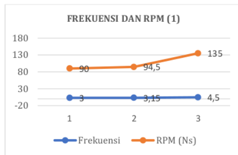
Gambar 7. Grafik Pengujian Frekuensi dan RPM Konveyor 1
