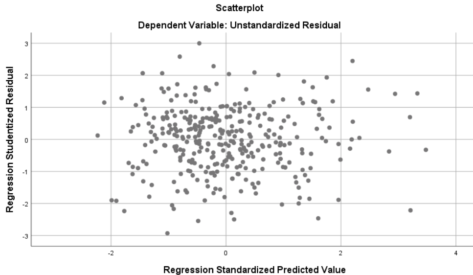
Gambar 1 Uji Heteroskedastisitas
