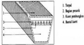
Gambar 2.1kontruksi V - Belt
