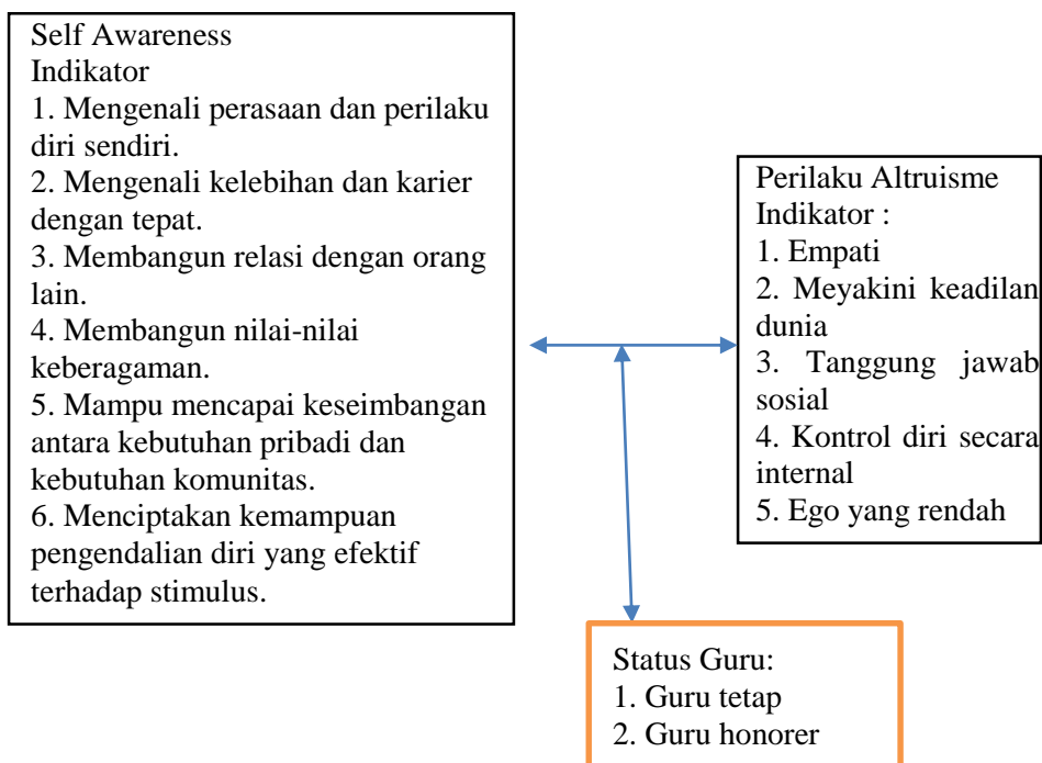
Gambar 1 Kerangka Berpikir
