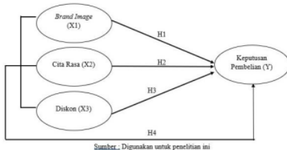
Gambar 2 Kerangka Pemikiran
