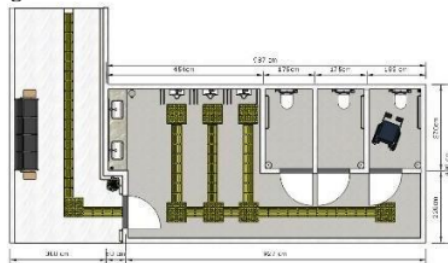
Gambar 5. Denah toilet disabilitas. (Sumber: Rancangan penulis)
