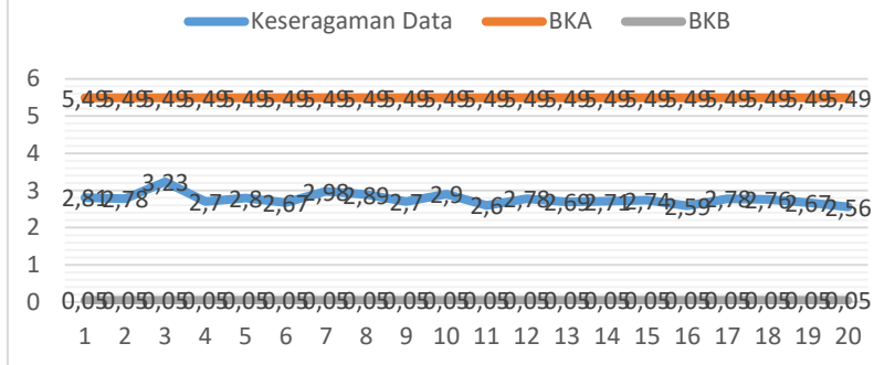
Lampiran 19 Batas Kontrol Sepatu PDH Doff
