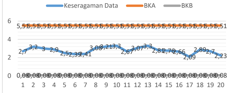
Lampiran 20 Batas Kontrol Sepatu PDH Doff
