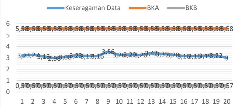
Lampiran 23 Batas Kontrol Sepatu PDH Doff
