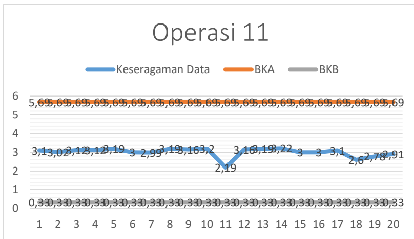
Lampiran 26 Batas Kontrol Sepatu PDH Doff
