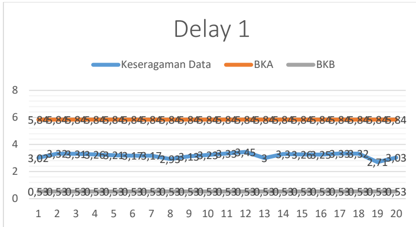
Lampiran 31 Batas Kontrol Sepatu PDH Doff
