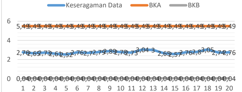
Lampiran 28 Batas Kontrol Sepatu PDH Doff
