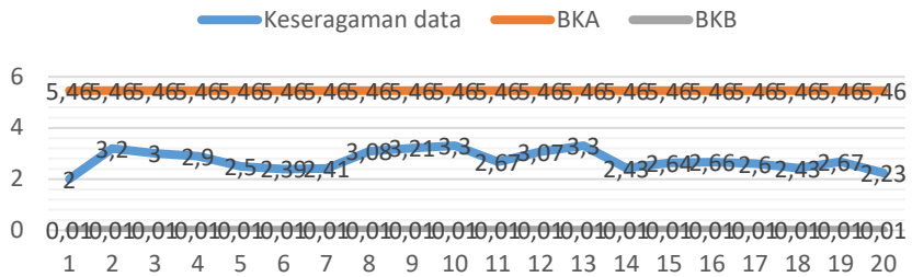
Lampiran 4 Batas Kontrol Sepatu PDH Kilap
