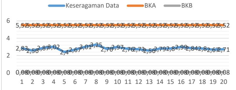
Lampiran 13 Batas Kontrol Sepatu PDH Kilap
