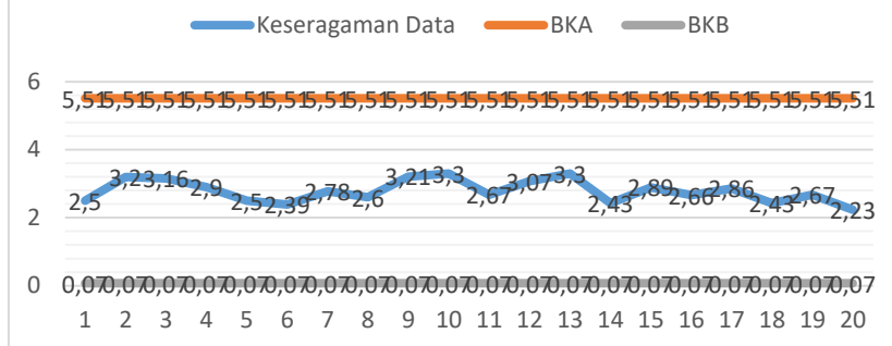
Lampiran 21 Batas Kontrol Sepatu PDH Doff
