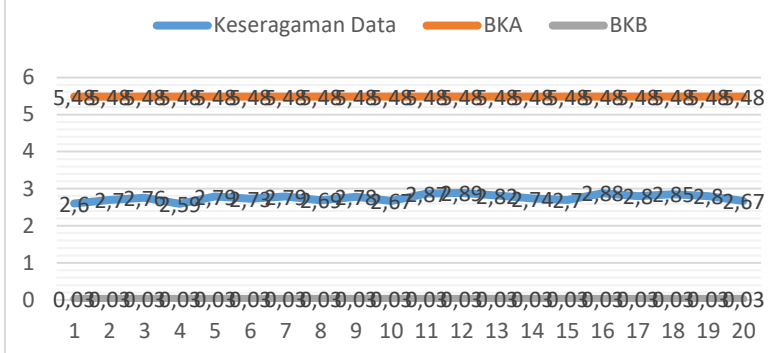
Lampiran 22 Batas Kontrol Sepatu PDH Doff
