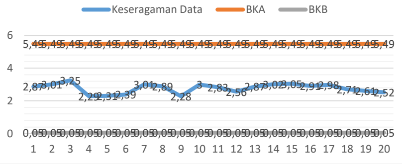
Lampiran 14 Batas Kontrol Sepatu PDH Kilap
