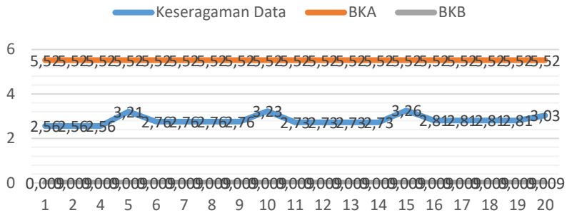
Lampiran 16 Batas Kontrol Sepatu PDH Kilap
