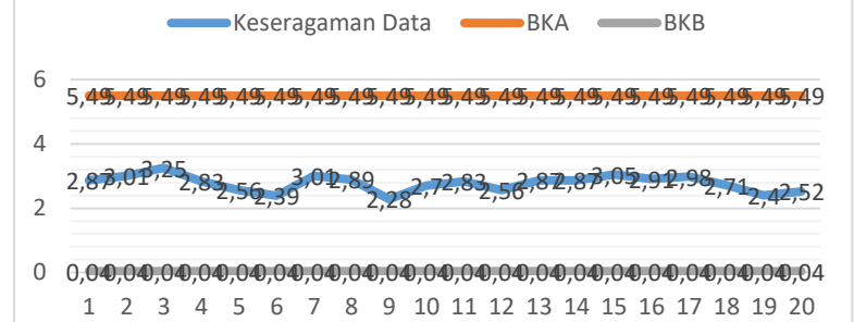
Lampiran 30 Batas Kontrol Sepatu PDH Doff
