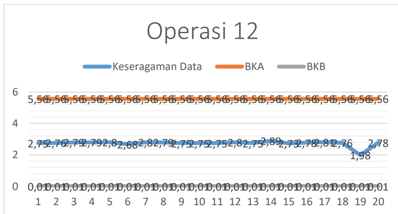
Lampiran 27 Batas Kontrol Sepatu PDH Doff
