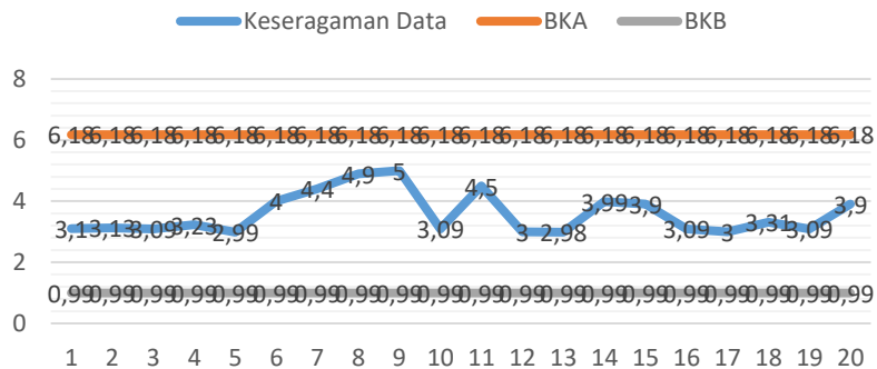
Lampiran 18 Batas Kontrol Sepatu PDH Doff
