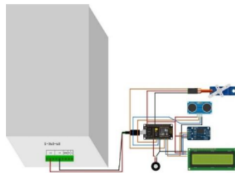
Figure 11. Rangkaian Keseluruhan
