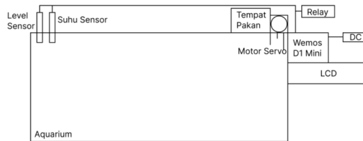
Figure 9. Desain Keseluruhan
