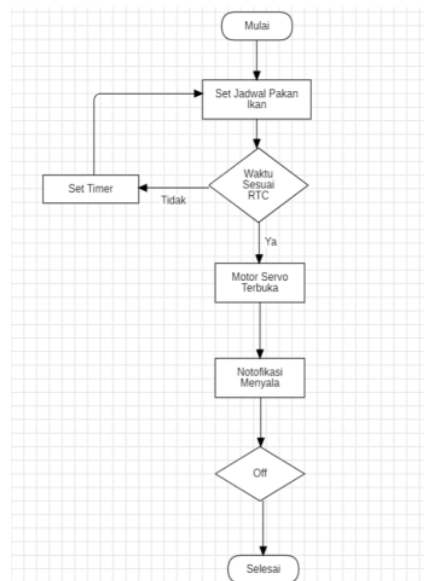
Figure 2. Alur Sistem Pemberi Pakan Ikan Otomatis
