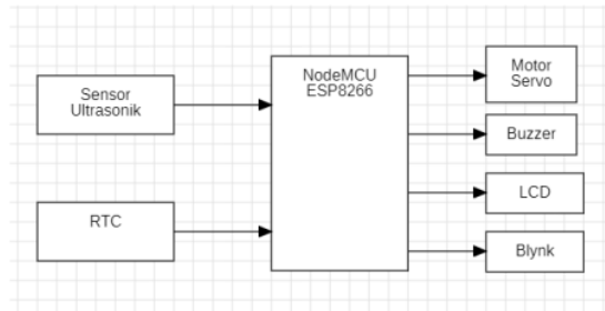
Figure 3. Blok Diagram Pemberi Pakan Ikan Otomatis
