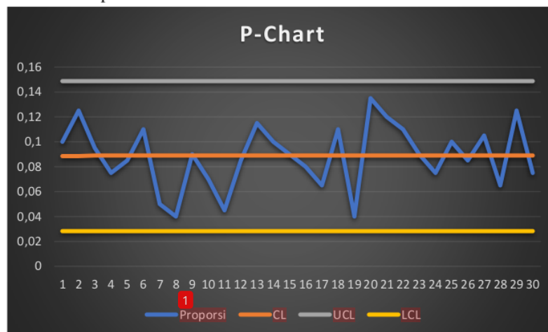
Gambar 2 Grafik P-Chart
