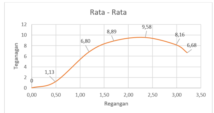
Gambar 21 grafik rata-rata tegangan regangan elektroda 1mm Arus 110A
