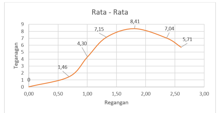
Gambar 20 grafik rata-rata tegangan regangan elektroda 1mm Arus 100A
