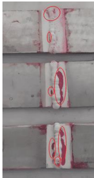
Gambar 7 hasil uji penetrasi elektroda diameter 0,8 dengan arus 100A
