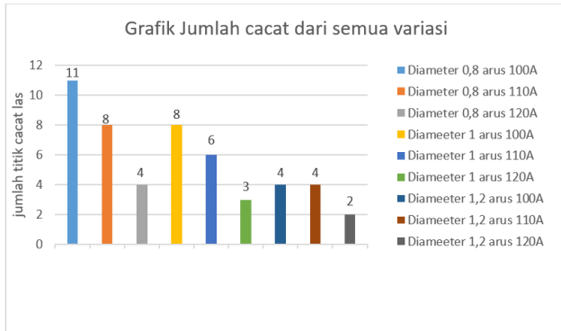
Gambar 15 jumlah keseluruhan cacat las
