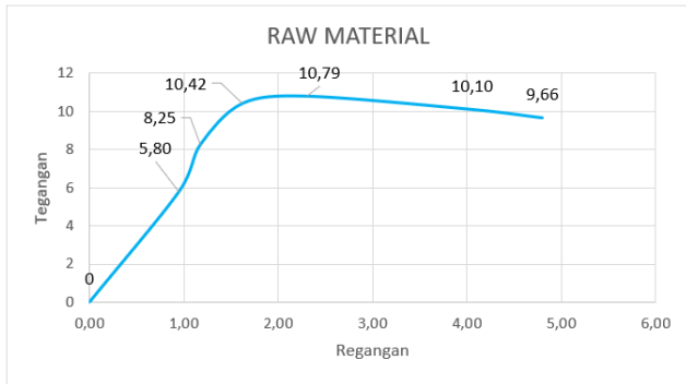
Gambar 16 Nilai tegangan regangan spesimen RAW
