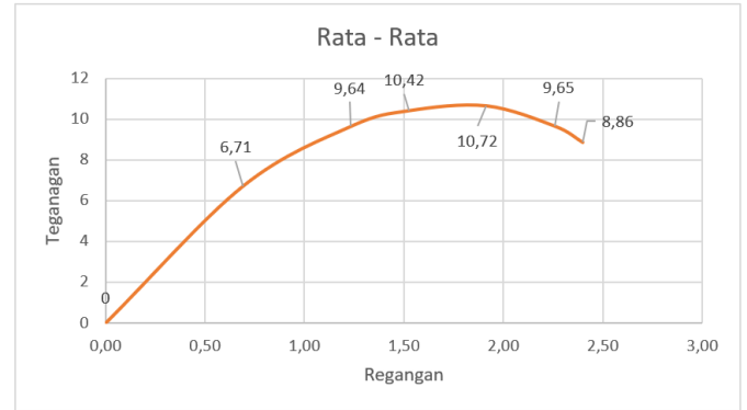
Gambar 24 grafik nilai rata-rata tegangan regangan elektroda 1,2mm Arus 120A
