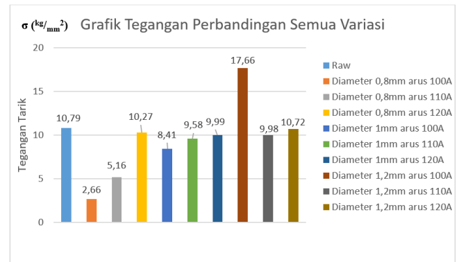
Gambar 25 grafik nilai tegangan dari semua variasi
