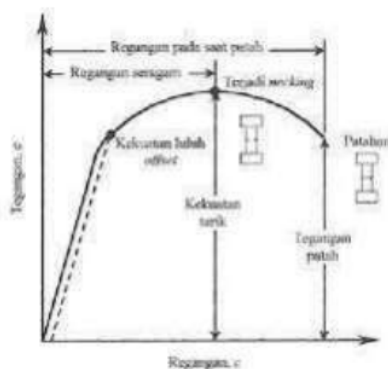
Gambar 2 . Proses Pengujian Tarik
