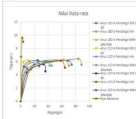
Gambar 3 Nilai rata-rata tegangan uji tarik.
