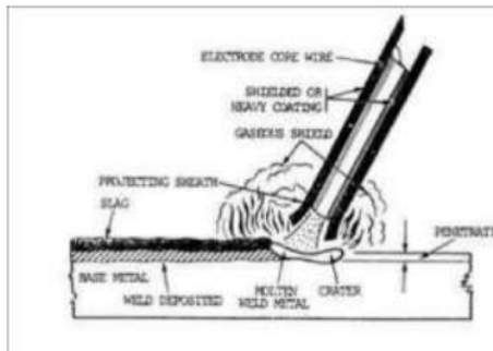
Gambar 1. Ilustrasi Proses Pengelasan SMAW
