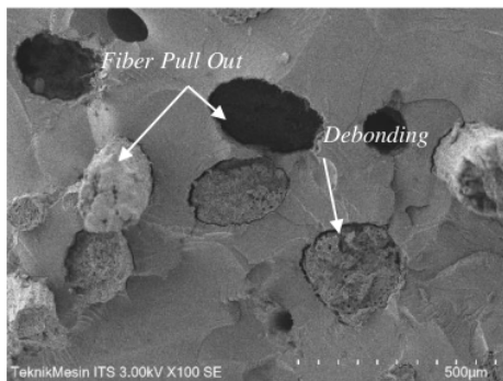
Gambar 20 Pengamatan SEM komposit fraksi volume 20 % rendaman 3 jam perbesaran x100
