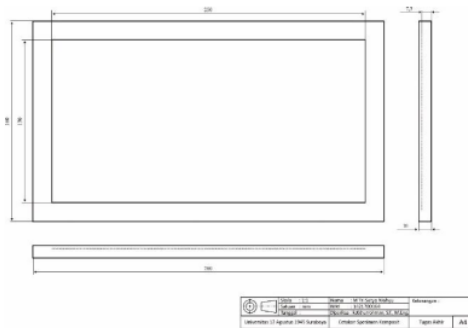
Gambar 13 ukuran cetakan
