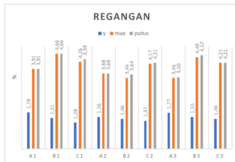
Gambar 18 Hasil Regangan Tarik
