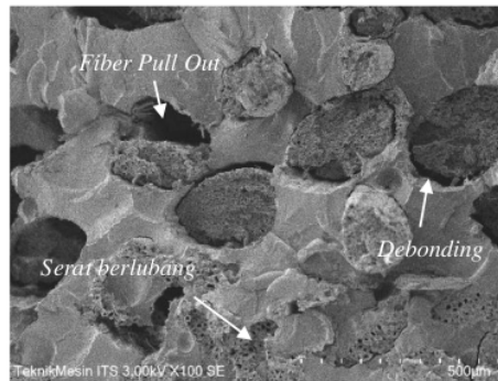
Gambar 21 Pengamatan SEM komposit fraksi volume 40 % rendaman 1 jam perbesaran x100
