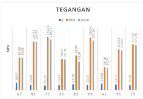
Gambar 17 Hasil Tegangan Tarik
