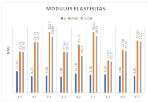
Gambar 19 Hasil Modulus Elastisitas
