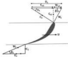
Gambar 10. Gambar Skema Segitiga Kecepatan
