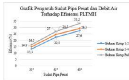
Gambar 12. Grafik Pengaruh Sudut Pipa Pesat dan Debit Air terhadap Efisiensi PLTMH
