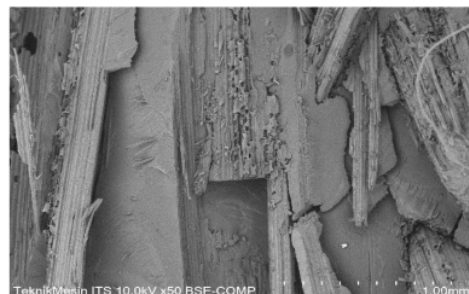
Gambar 14 Hasil Uji SEM Spesimen Tarik (B3.2) Perbesaran 50x
