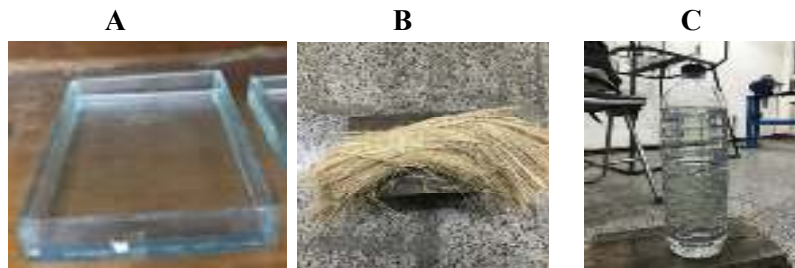
Keterangan : A. Cetakan Spesimen B. Serat Bambu Apus C. Resin Polyester
