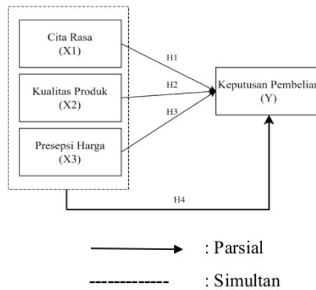
Gambar 1 Kerangka Konseptual
