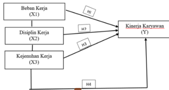
Gambar 1 Kerangka Konseptual
