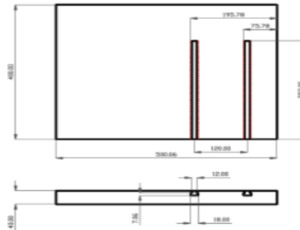
Gambar 13. Desain Alas
