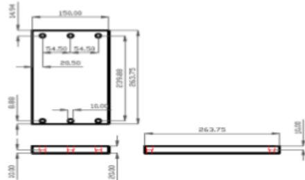
Gambar 12. Desain Batang Tiang Penghubung
