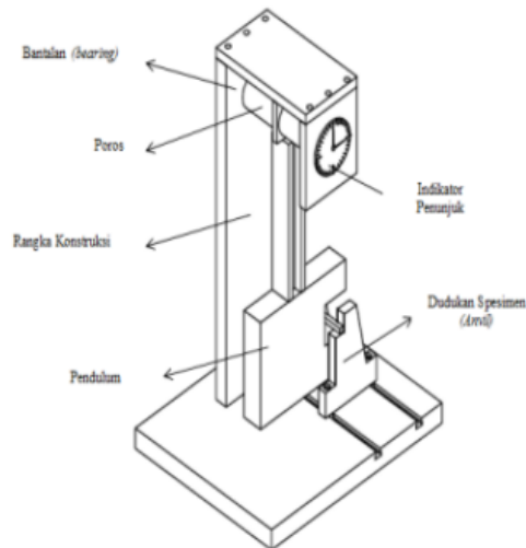
Gambar 2. Desain Mesin Uji Impact Charpy
