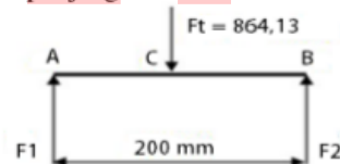
Gambar 6. Pembebanan pada bantalan
