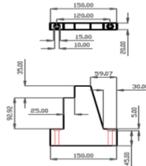
Gambar 14. Desain Dudukan Spesimen Uji
