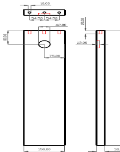
Gambar 10. Desain Batang Tiang Penahan I
