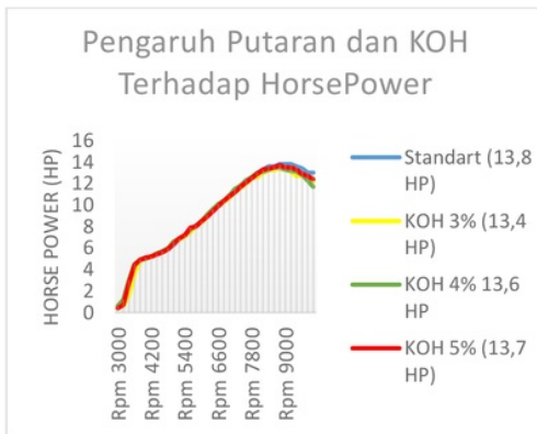
Grafik 1. Pengaruh Putaran dan Variasi KOH terhadap HorsePower
