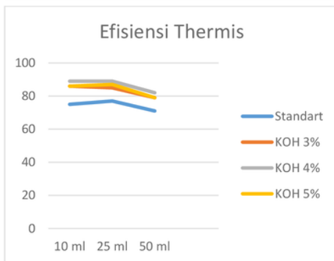
Grafik 6. Efisiensi Thermis
