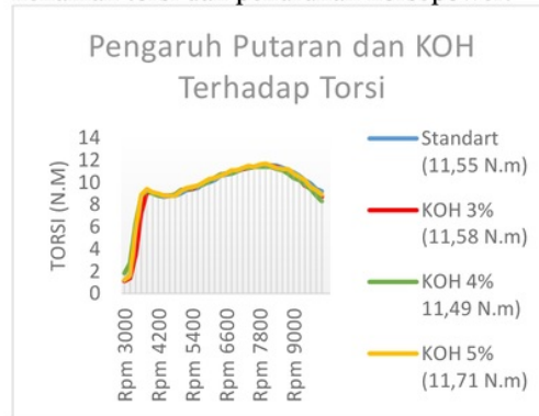
Grafik 2. Pengaruh Putaran dan Variasi KOH terhadap Torsi
