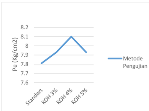
Grafik 3. Tekanan Efektif Rata Rata
