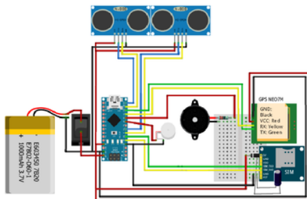
Gambar 3 Rancangan Komponen Elektronika
