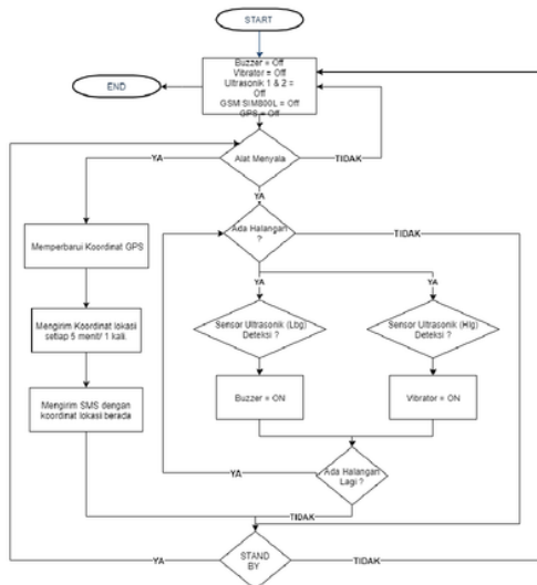
Gambar 2 Flowchart Perangkat Keras
