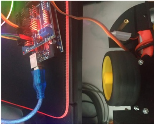
Gambar 3.5 Servo yang sudah dipasang roda
