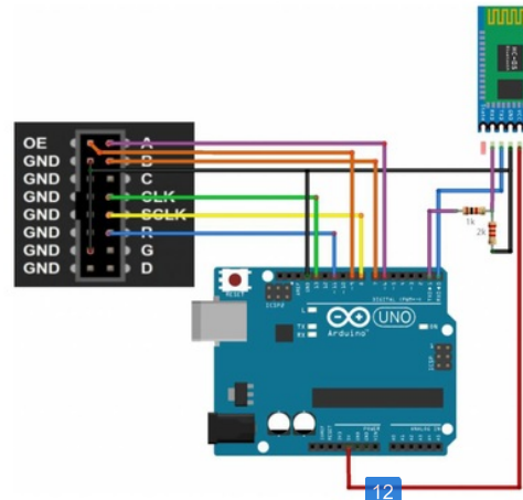
Gambar 2.7 Tampilan Input Arduino Uno Dengan Modul Bluetooth HC-05
