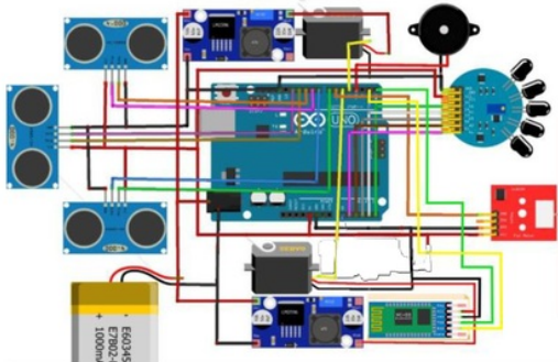
Gambar 2.8 Tampilan Rancangan Keseluruhan
