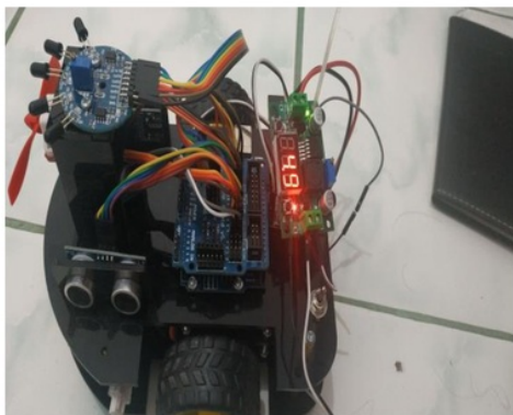
Gambar 3.11 Keseluruhan Rangkaian Robot Pencari Sumber Api
