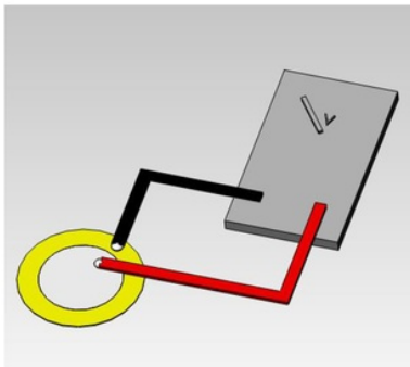
Gambar 2.2 Mekanisme piezoelektrik
