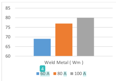
Gambar Grafik nilai rata-rata weld metal uji rockwell kampuh X
