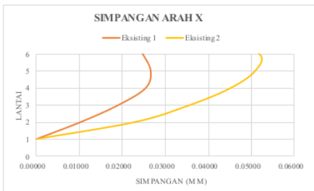
Gambar 4 1 Grafik Defleksi Arah X
