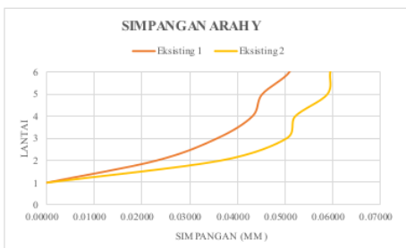
Gambar 4.2 Grafik Defleksi Arah Y
