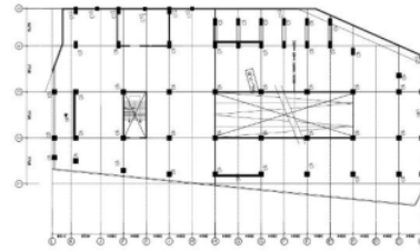
Gambar 3.1 Permodelan Dinding Geser Di tepi
