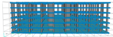
Gambar 3.4 Permodelan Struktur 3D
