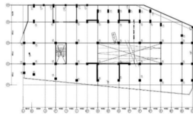
Gambar 3.3 Permodelan Dinding Geser Ditengah
