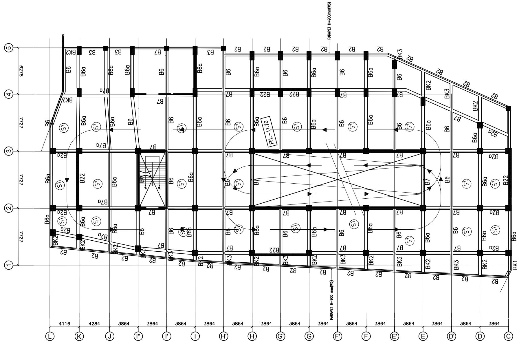
DENAH BALOK & PLAT LT BASEMENT 3-7 SKALA 1 : 100
