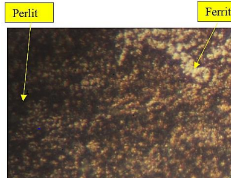
Gambar 17. Hasil pengujian struktur mikro spesimen Z
