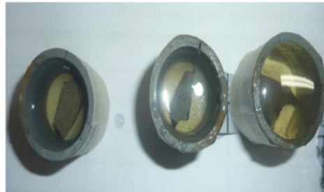
Gambar 10. Spesimen dalam cetakan
