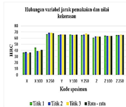
Gambar 18. Hubungan variabel jarak pemakaian dan nilai pengujian kekerasan rockwell
