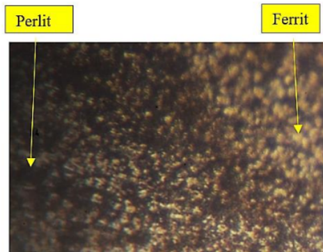
Gambar 16. Hasil pengujian struktur mikro spesimen Y
