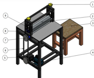
Gambar 8. Usulan Rancangan Alat Pengerol Sendal
