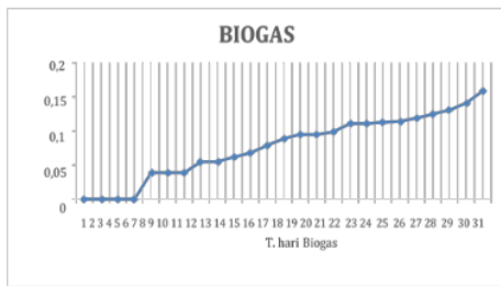
Gambar 11. Grafik laju hasil biogas
