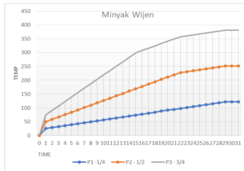
Gambar 7. Pengaruh waktu dan tekanan terhadap titik didih minyak wijen
