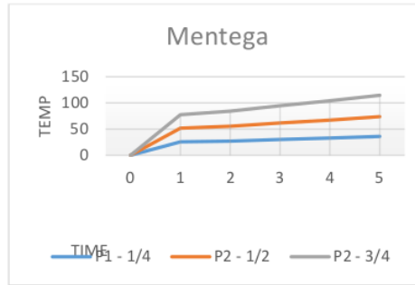
Gambar 10. Pengaruh waktu dan tekanan terhadap titik didih mentega
