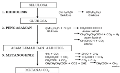
Gambar 3 Tahap proses pembuatan Biogas
