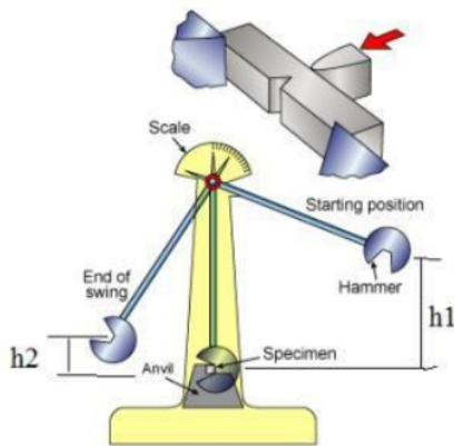
Simulasi kerja pengujian impak
