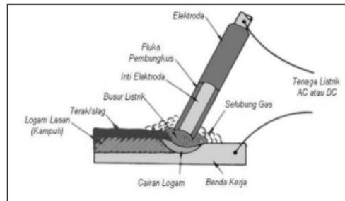
Ilustrasi Las SMAW
