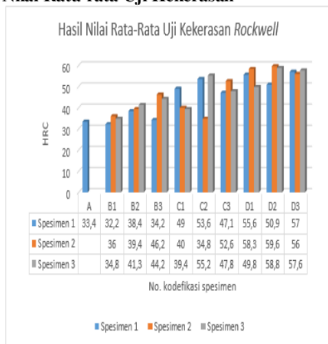
Gambar 8. Diagram Rata-rata Nilai Kekerasan per Spesimen
