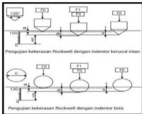
Gambar 4. Skema Uji Kekerasan Rockwell
