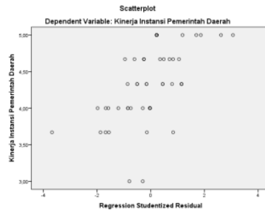
Gambar 2 Uji Heteroskedastisitas
