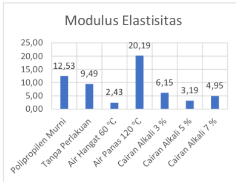
Gambar 15. Grafik Modulus Elastisitas terhadap dengan 6 varian perlakuan
