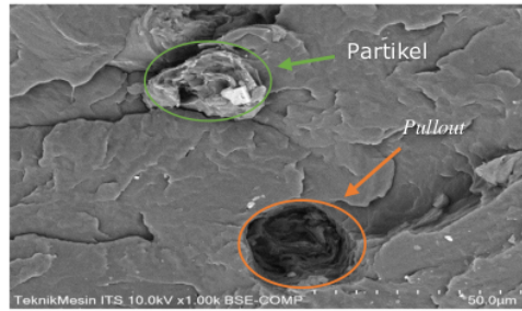
Gambar 18. Morfologi Sampel Uji Tarik Max Perlakuan Variasi Cairan Alkali 7% Zoom 1000x
