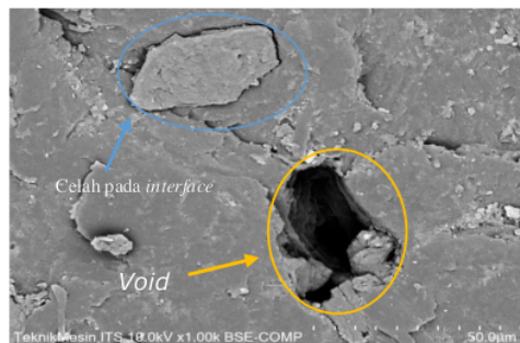
Gambar 22. Morfologi Sampel Uji Tarik Max Perlakuan Variasi Air Panas 120°C Zoom 1000x
