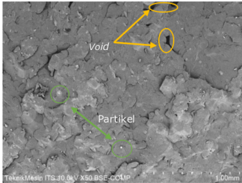
Gambar 17. Morfologi Sampel Uji Tarik Max Perlakuan Variasi Cairan Alkali 7% Zoom 50x
