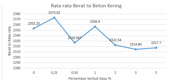
Gambar 5. Grafik Rata-rata Berat Isi Beton Kering
