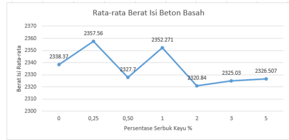
Gambar 4. Grafik Rata-rata Berat Isi Beton Basah
