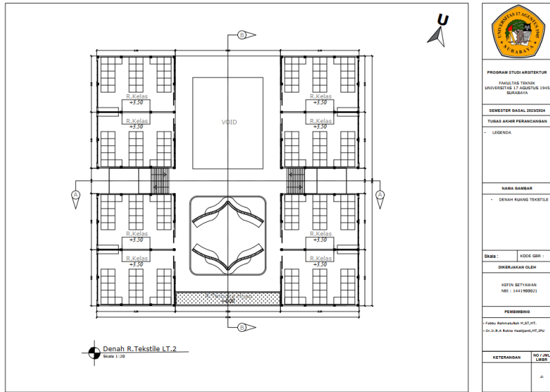
Gambar 6.2.7 Denah Ruang Tekstile
