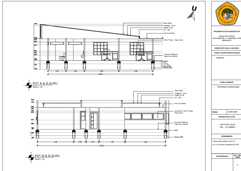
Gambar 6.2.15 Potongan Ruang Guru
