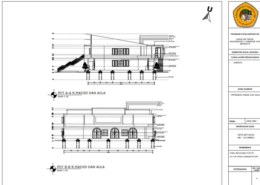
Gambar 6.2.12 Potongan Masjid dan Aula
