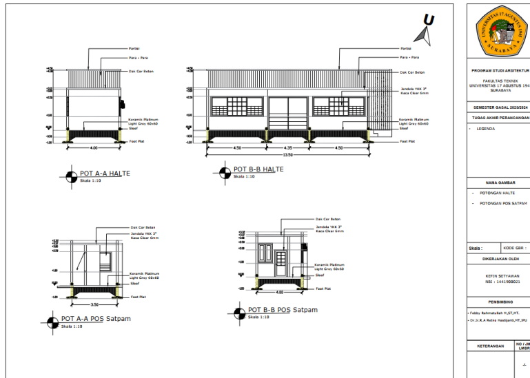
Gambar 6.2.18 Potongan Halte dan Pos Satpam
