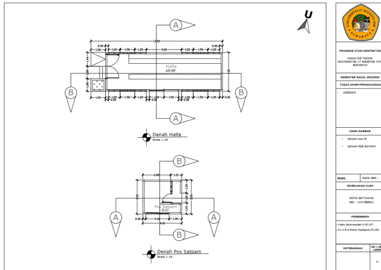
Gambar 6.2.17 Denah Halte dan Pos Satpam
