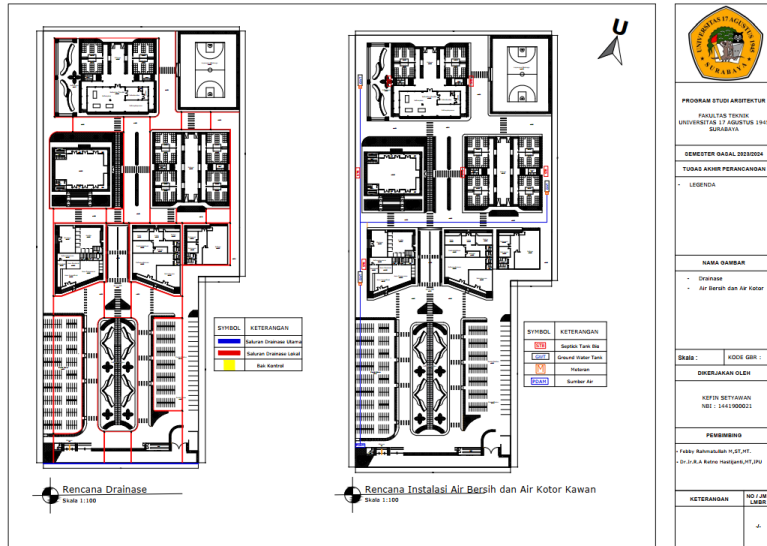
Gambar 6.3.2 Rencana Drainase Air Bersih dan Air Kotor
