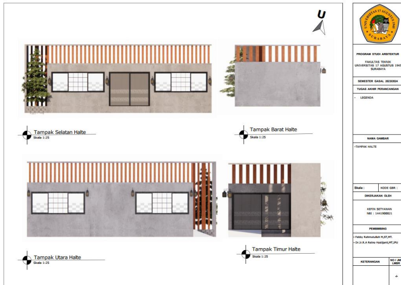
Gambar 6.2.19 Tampak Halte
