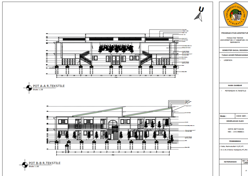
Gambar 6.2.8 Potongan Ruang Tekstile
