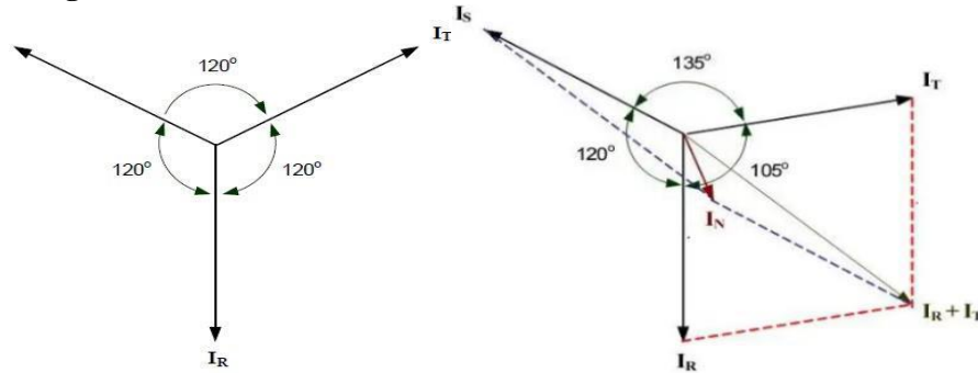
Gambar 2. Diagram Vektor Beban Seimbang dan Tidak Seimbang
