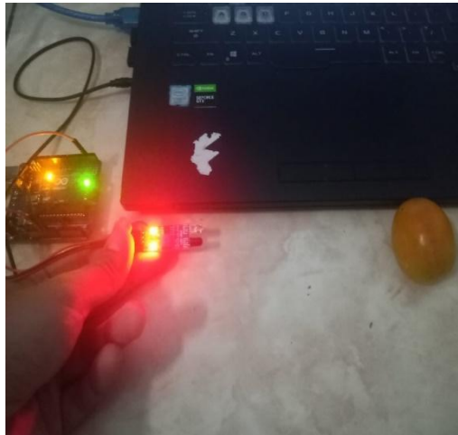
Gambar 5. Gambar Pengujian Sensor Inframerah
