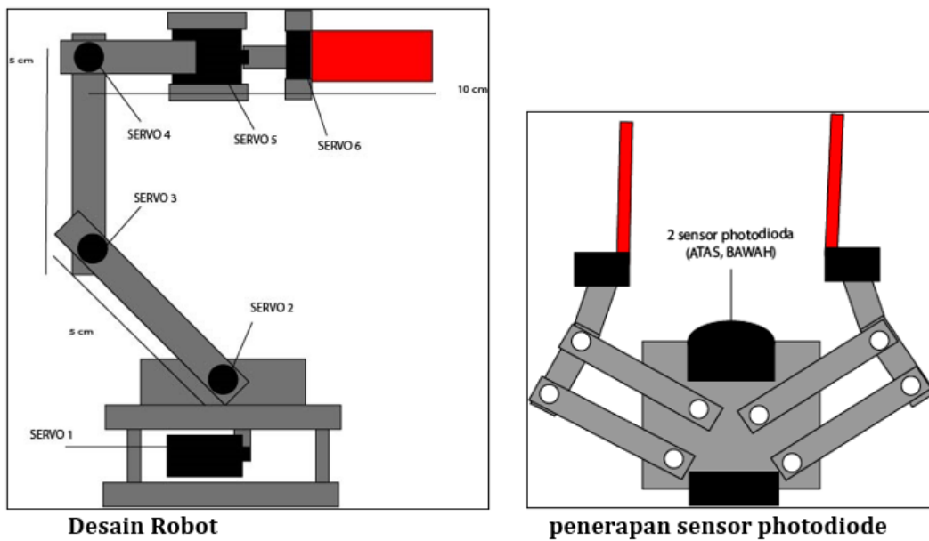
Gambar 3. Desain Robot Lengan
