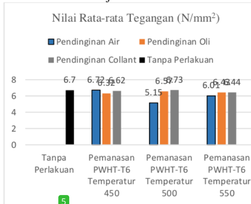
Gambar 3 Nilai rata-rata tegangan uji tarik.
