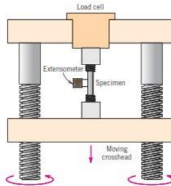
Gambar 1. Ilustrasi mesin pengujian Tarik.
