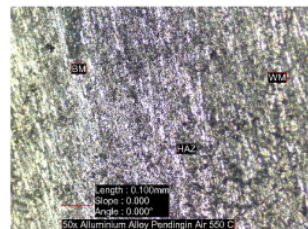
Gambar 7. Hasil mikro temperatur pemanasan 550 dengan media pendinginan air.
