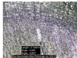
Gambar 6. Hasil mikro temperatur pemanasan 500 dengan media pendinginan air.
