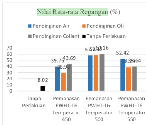
Gambar 4 Nilai rata-rata regangan uji tarik.
