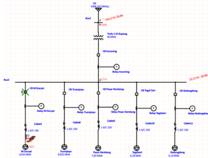
Gambar 5. Simulasi OCR Menggunakan Etap 19.0.1
