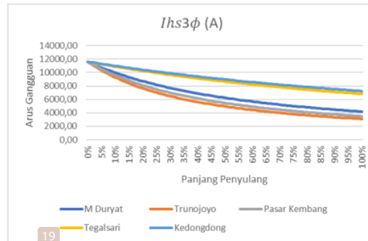
Gambar 2. Arus Hubung Singkat 3 Fasa Pada Setiap Penyulang
