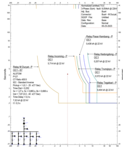
Gambar 6. Kurva TCC OCR Hasil Simulasi
