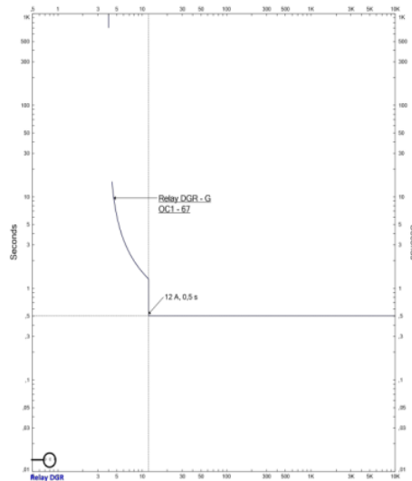
Gambar 7. Kurva TTC DGR Hasil Simulasi
