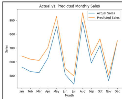
Gambar 9. Grafik Perbandingan Data Penjualan Aktual dan Prediksi
