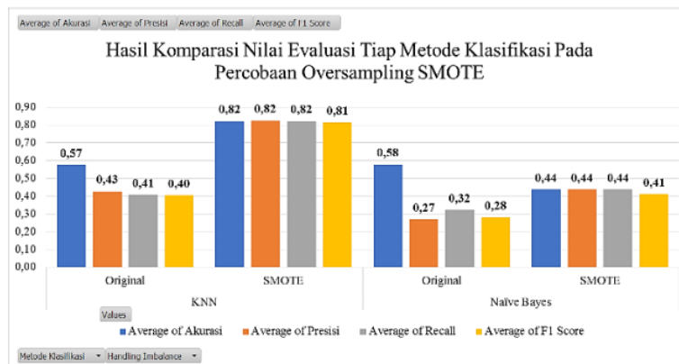
Gambar 7. Hasil Komparasi Nilai Evaluasi Metode KNN dan Naive Bayes Pada Uji Coba Teknik Oversampling SMOTE
