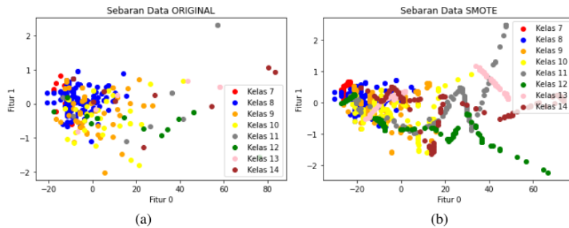
Gambar 4. Plot Perbandingan Sebaran (a) Data Original dan (b) Data Synthetic Pada Uji Coba 8 Kelas Klasifikasi dengan Pengambilan 100 Data
