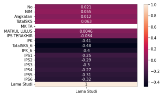
Gambar 2. Uji Korelasi Seluruh Variabel Terhadap Lama Studi Mahasiswa 8 Kelas
