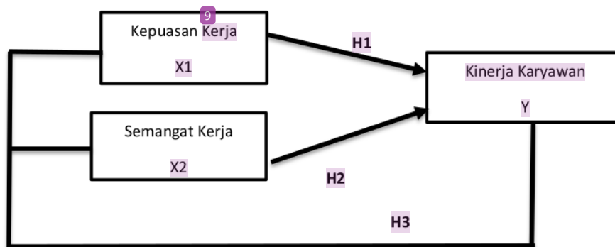
Gambar 2.2 Kerangka Konseptual
