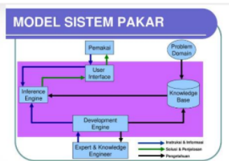
Gambar 2. 1 Sistem Pakar
