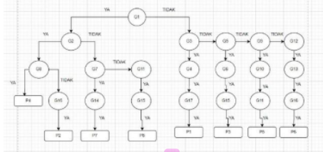
Gambar 3. 1 Pohon Keputusan
