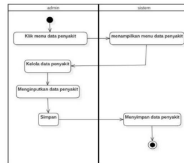
Gambar 2. 4 Activity diagram menambah penyakit
