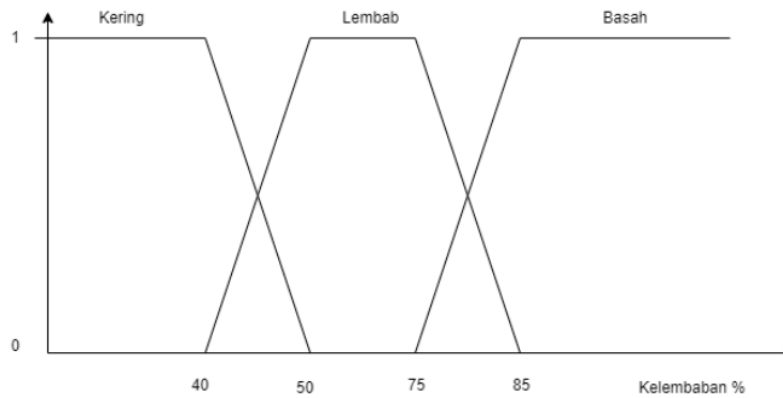
Gambar 9. Fungsi Keanggotaan Sensor Kelembapan 1
