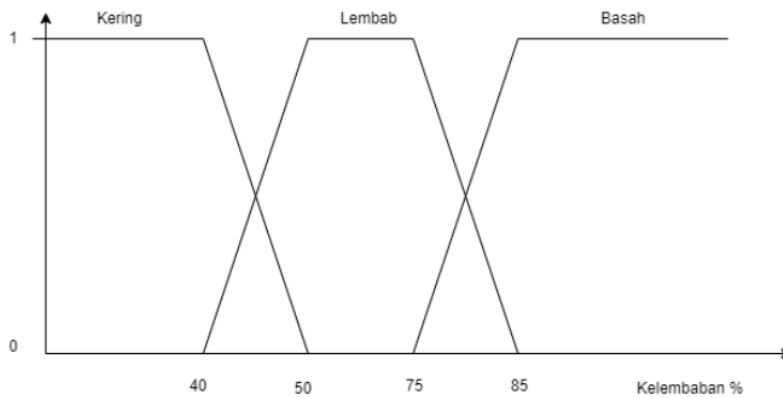
Gambar 10. Fungsi Keanggotaan Sensor Kelembapan 2
