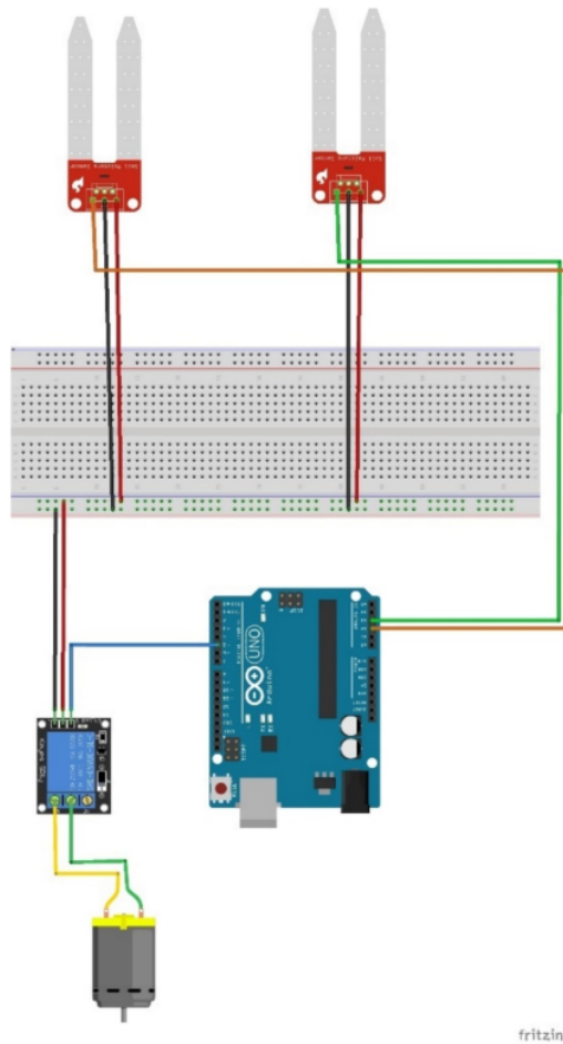
Gambar 3. Rangkaian Elektronika
