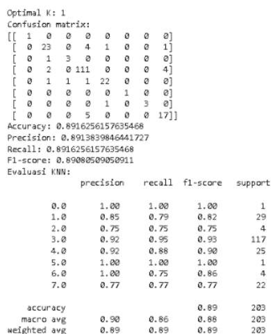
Gambar 9. Hasil Akurasi K=1
