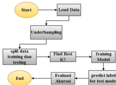
Gambar 4. Klasifikasi KNN
