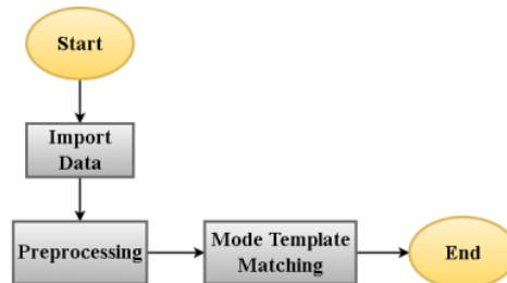
Gambar 3. Template Matching
