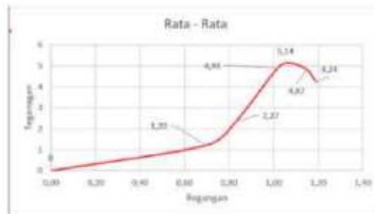
Gambar 18 grafik rata-rata tegangan regangan elektroda 0,8 dengan Arus 100A
