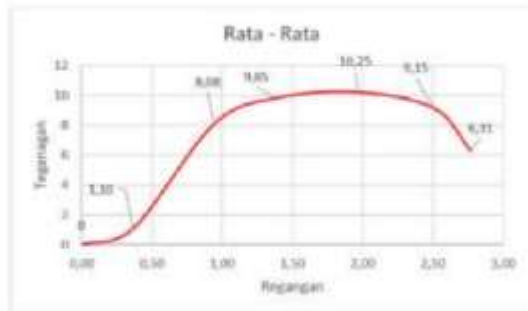
Gambar 24 grafik rata-rata tegangan regangan elektroda 1,2mm dengan Arus 120A
