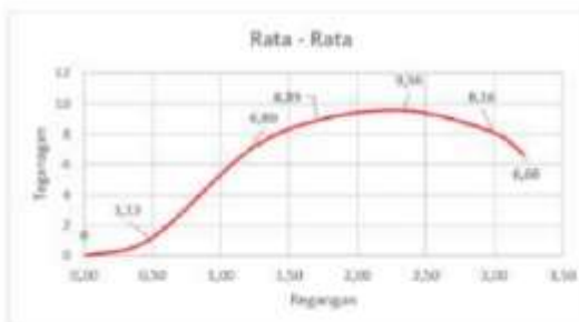
Gambar 23 grafik rata-rata tegangan regangan elektroda 1,2mm dengan Arus 100A
