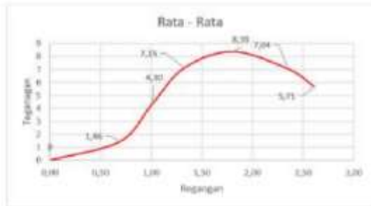
Gambar 20 grafik rata-rata tegangan regangan elektroda 1mm dengan Arus 80A
