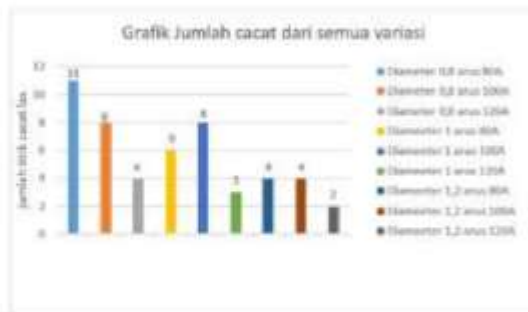
Gambar 15 grafik jumlah cacat dari semua variasi
