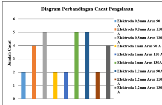
Gambar 16. Diagram Jumlah Cacat Setiap Variasi
