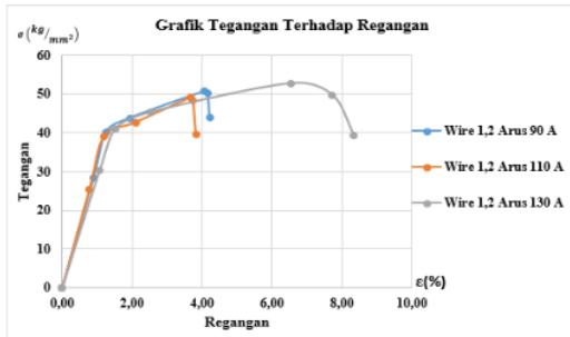
Gambar 23. Grafik Rata-Rata Tegangan dan Regangan Variasi Diameter Wire Ø1,2 Arus 90A, 110A, 130A
