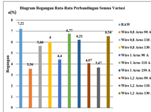
Gambar 25. Diagram Regangan Rata-rata Semua Variasi
