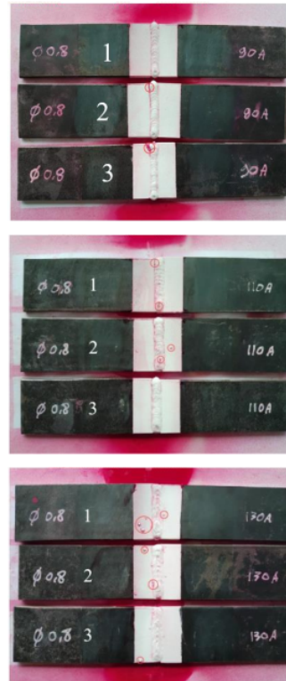
Gambar 13. Penetran Variasi Wire Ø0,8 Arus 90A, 110A, 130A
