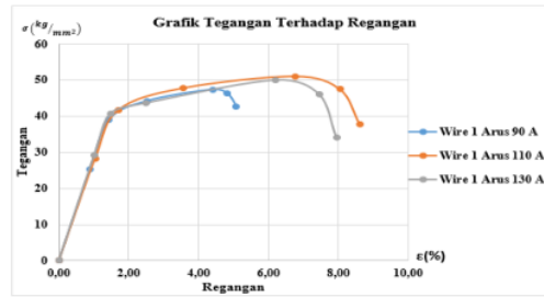
Gambar 21. Grafik Rata-Rata Tegangan dan Regangan Variasi Diameter Wire Ø1 Arus 90A, 110A, 130A
