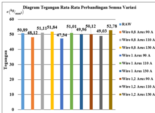
Gambar 24. Diagram Tegangan Rata-rata Semua Variasi
